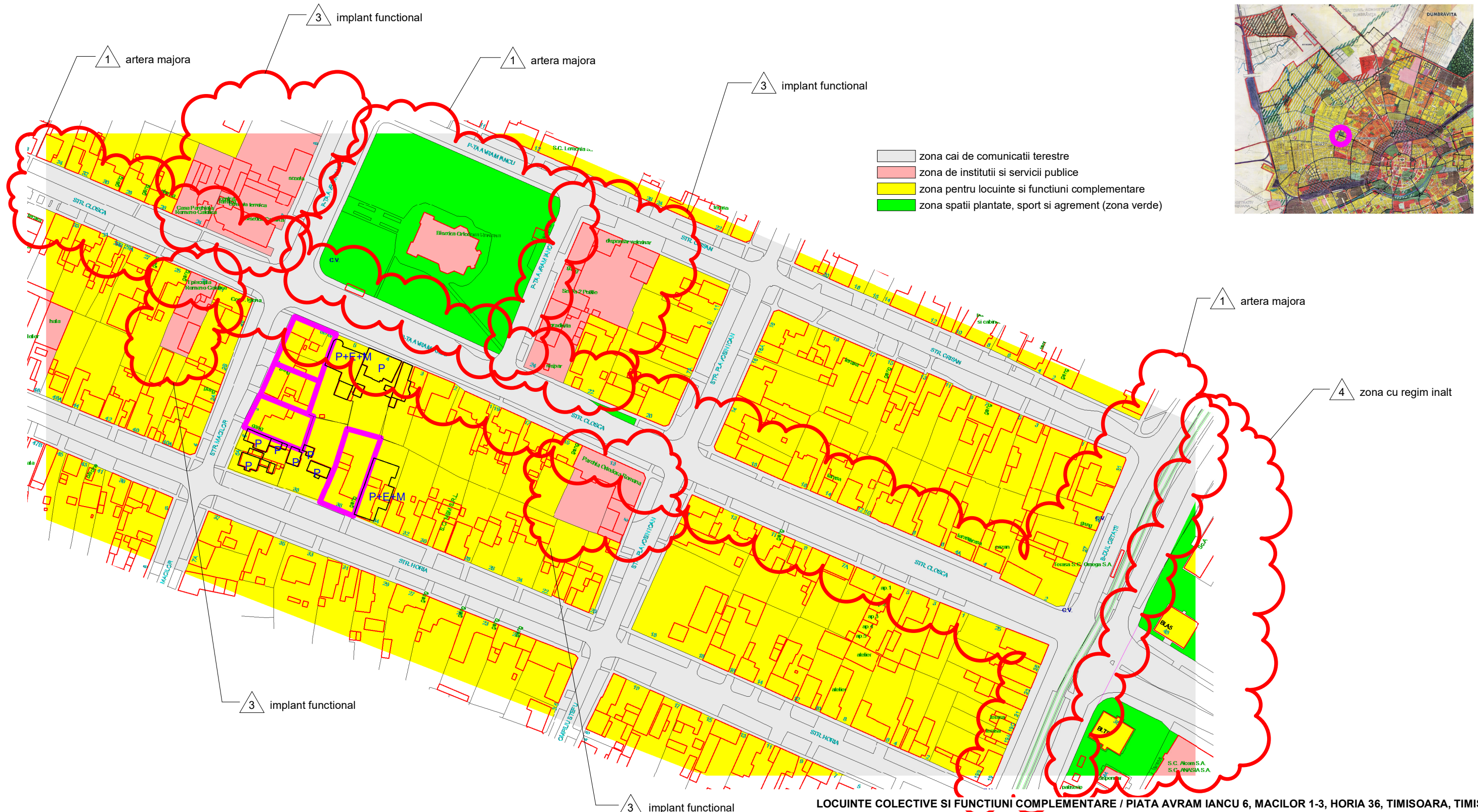
1 plan de situatie existent cvartal 1 : 2000
